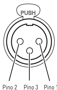
Conector de entrada equalizado (XLR fêmea)
