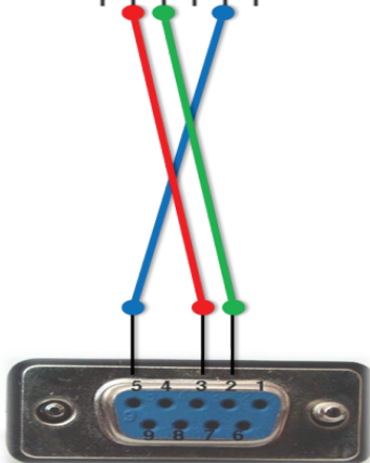
DB9 femelle – Vue de face du connecteur
